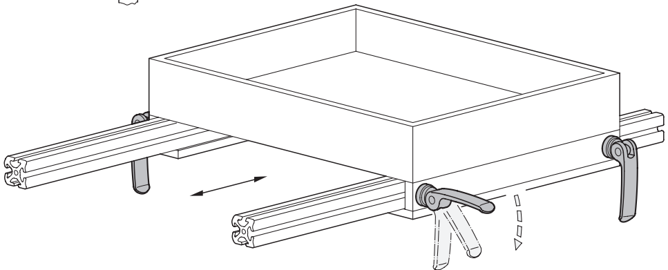
货架托盘或 存储托盘等 支持线型调整
