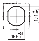
钻孔模板
