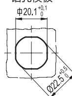
钻孔模板
