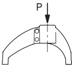
最大静载荷 P = 9800 \text{ N}
