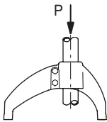
连接件保持力 P = 2000 \text{ N}
